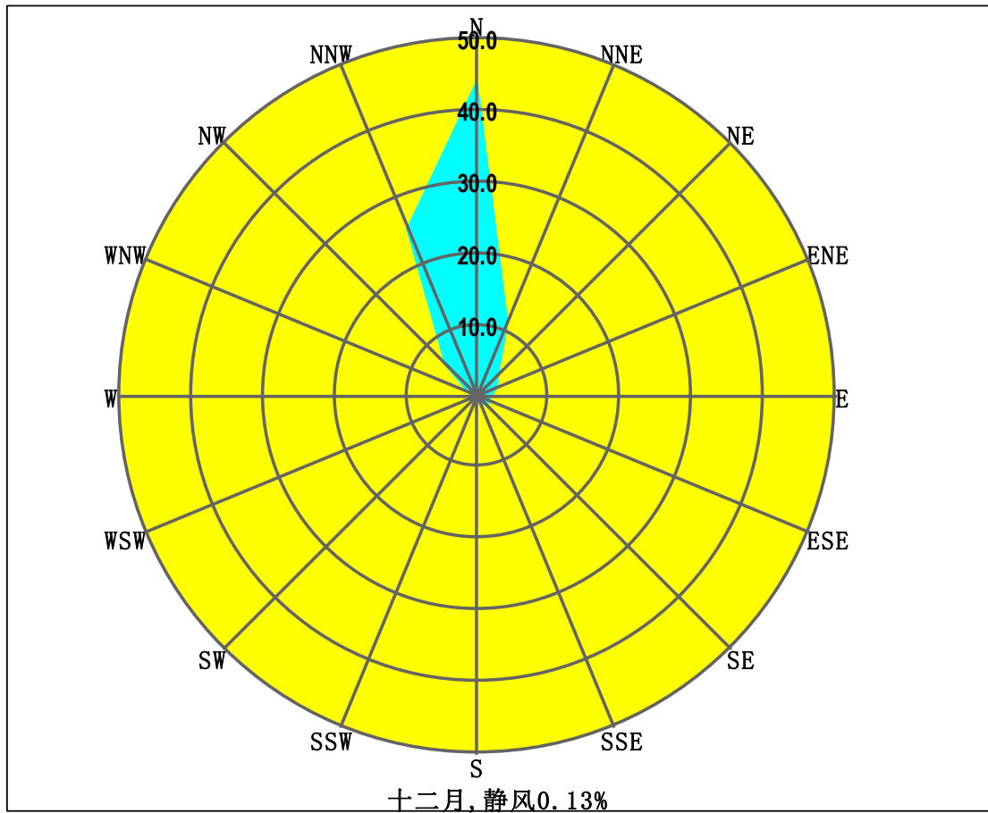
图3 广州(黄埔)国家基本气象观测站 2016年12月份16方位逐时风频玫瑰图
