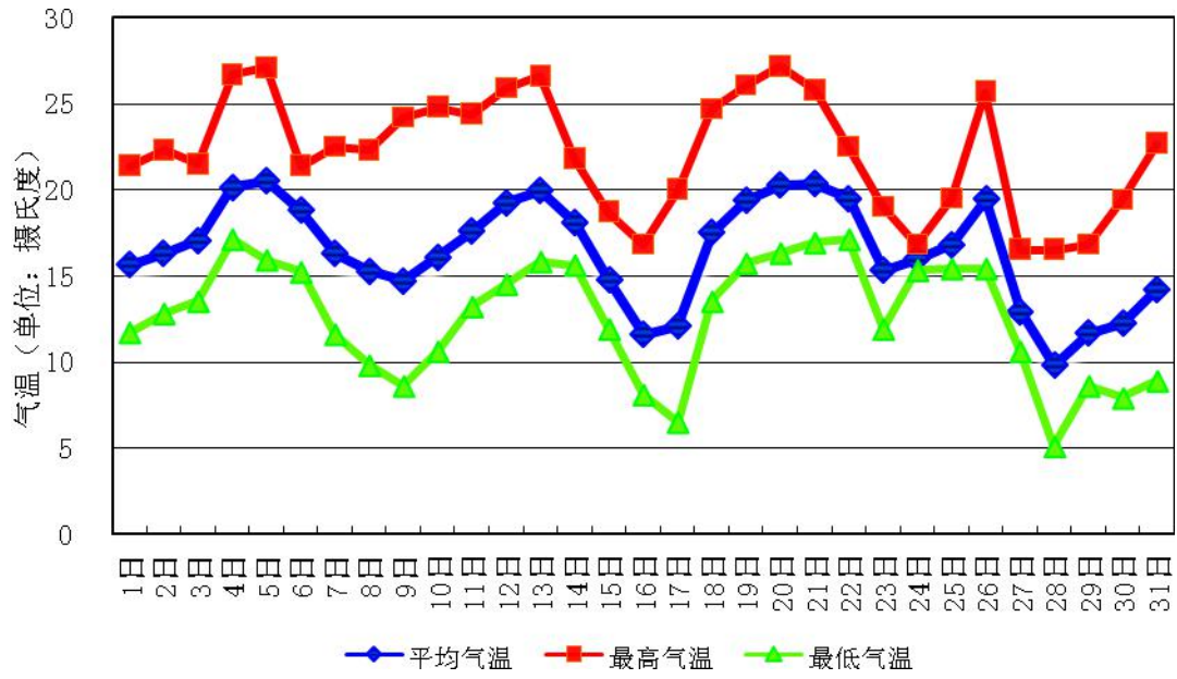
图 1 广州(黄埔)国家基本气象观测站 2016 年 12 月份逐日气温曲线
