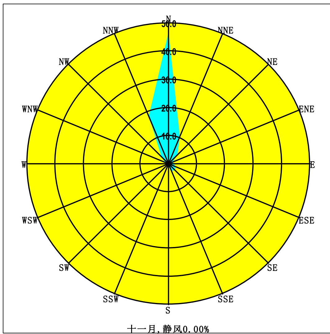
图3 广州(黄埔)国家基本气象观测站 2016 年 11 月份 16 方位逐时风频玫瑰图
