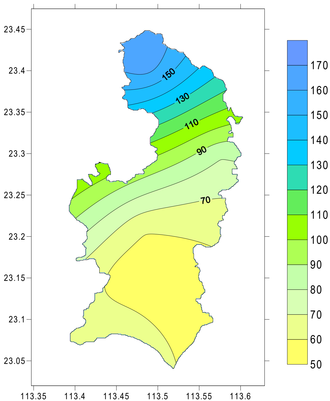
图 4 黄埔区 2016 年 11 月降水分布图（单位：毫米）
