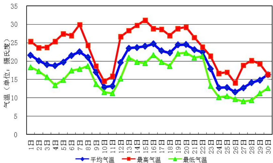
图 1 广州(黄埔)国家基本气象观测站 2016 年 11 月份逐日气温曲线
