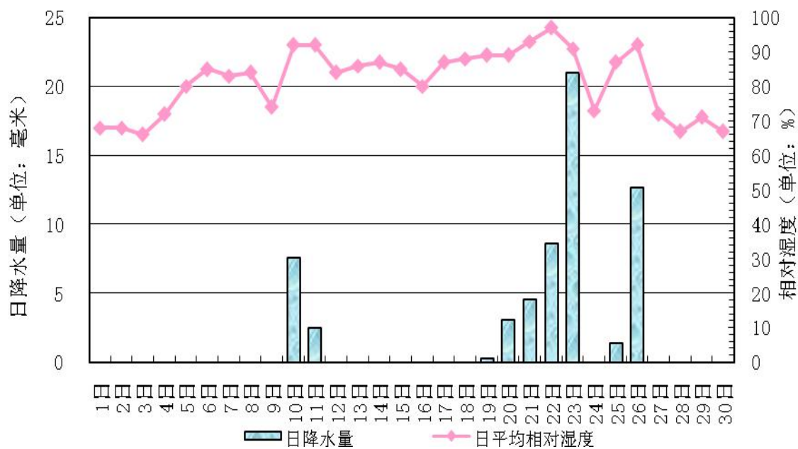
图 2 广州(黄埔)国家基本气象观测站 2016 年 11 月份逐日湿度和降水量曲线
