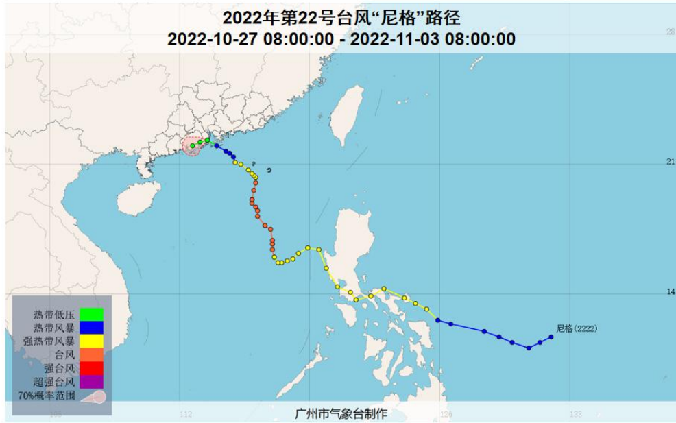
图 1 2022 年第 22 号台风“尼格”路径图
