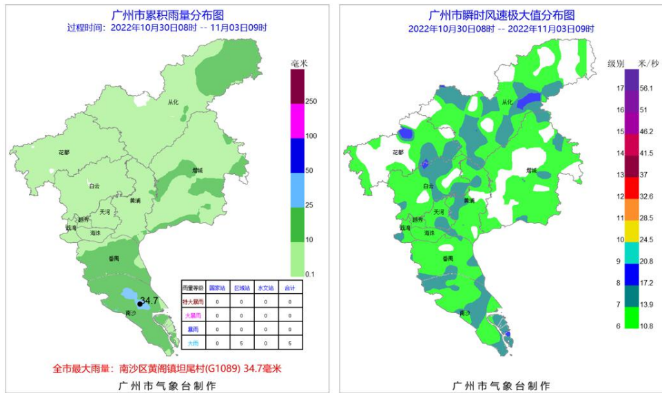
图 2 2022 年 10 月 30 日 08 时至 11 月 3 日 09 时广州市过程累积雨量（单位：毫米） 和极大风速（单位：米/秒）
